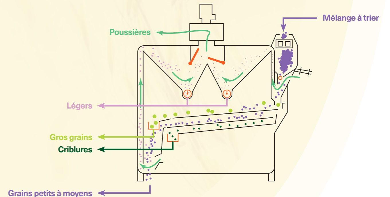
Figure 19 • Schéma légendé du trieur SVD 100
